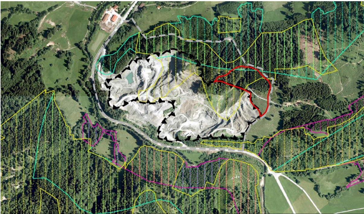
Waldfunktionskartierung
